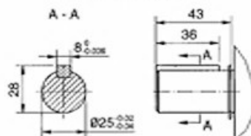
平键 Plain key
